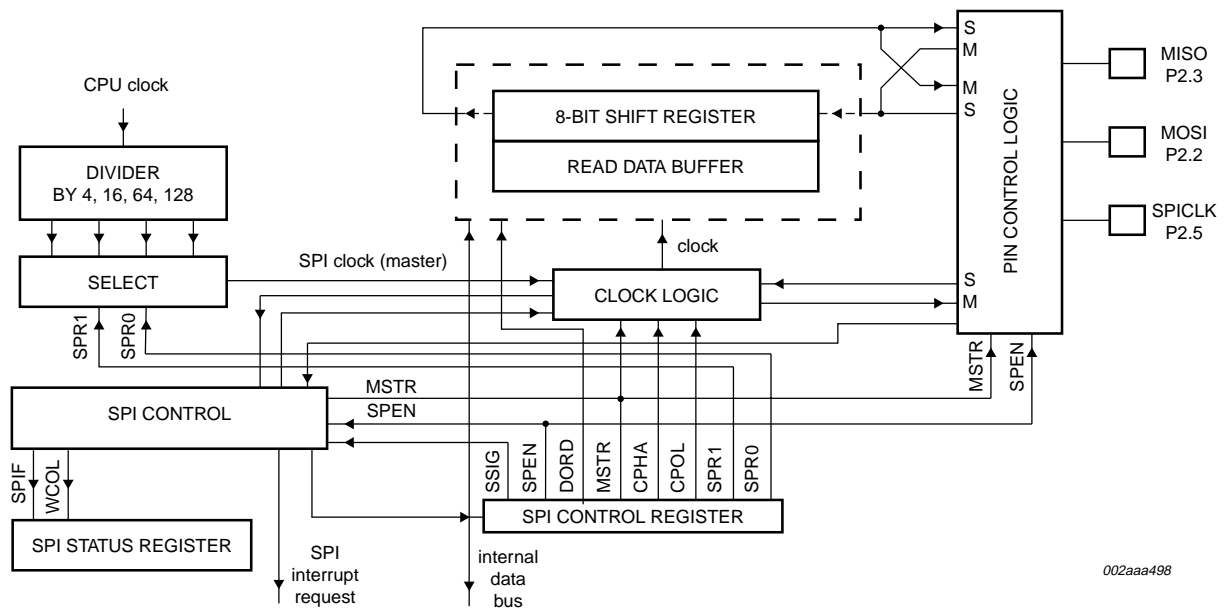
Fig 17. SPI block diagram (P89LPC913).
